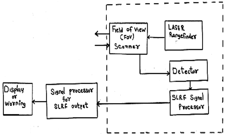
આકૃતિ-૨: લેઝર રેન્જ ફાઈન્ડર વાયર વોર્નિંગ પ્રણાલી કાર્યપદ્ધતિ
